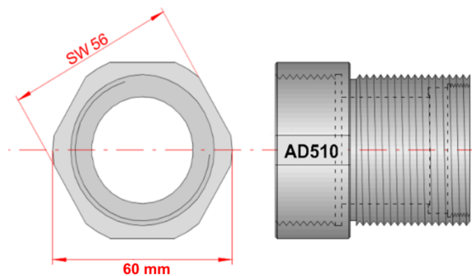
Fig. 3 Adapter AD510
